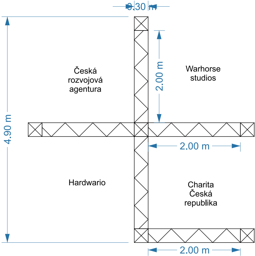
Půdorys:
